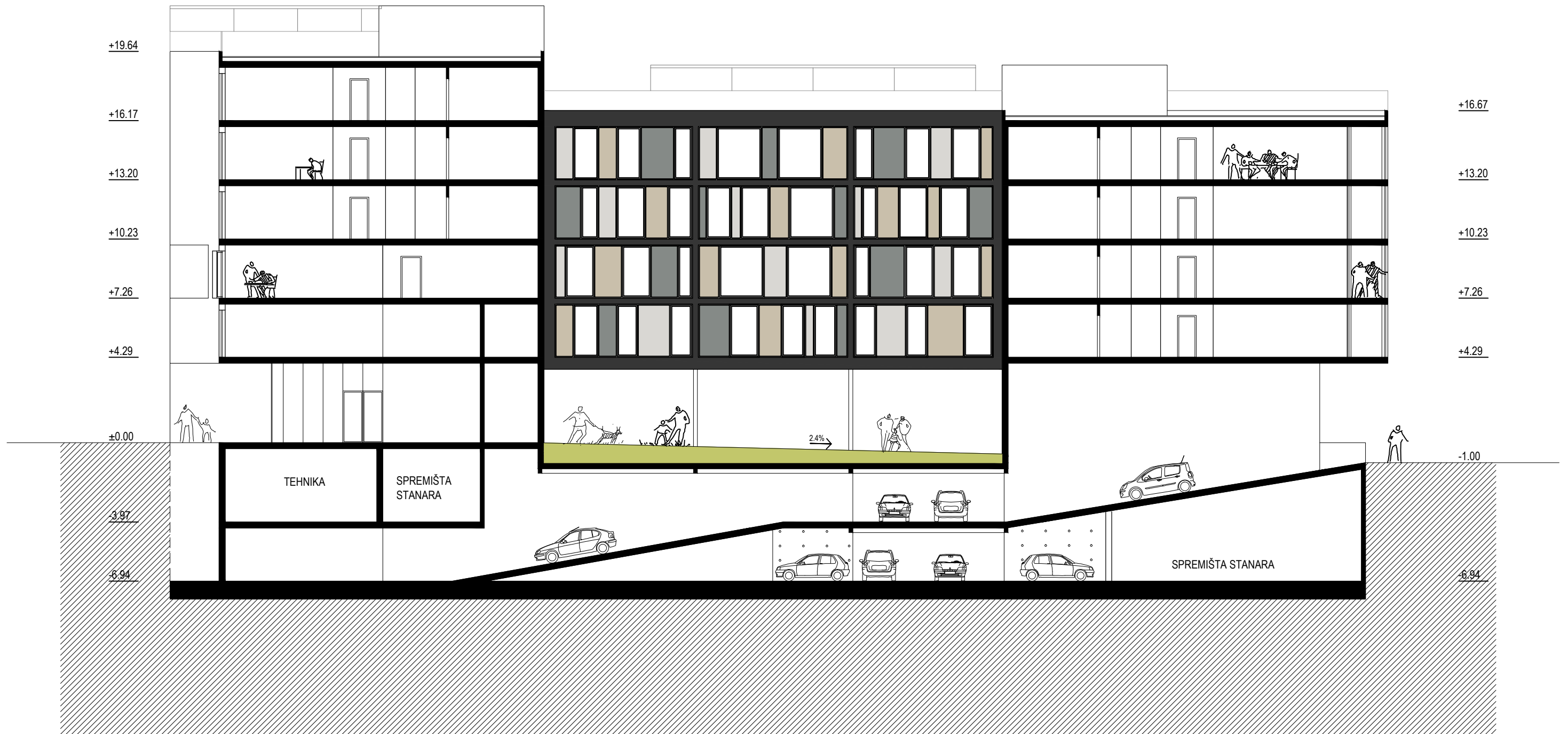
PRESJEK A-A
